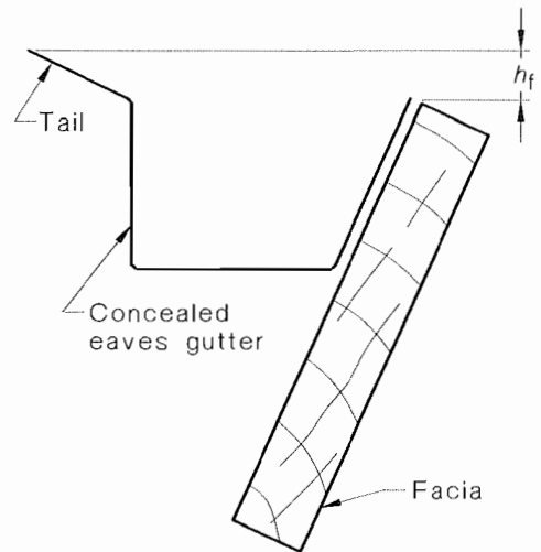
(d) Concealed eaves gutter with tail
